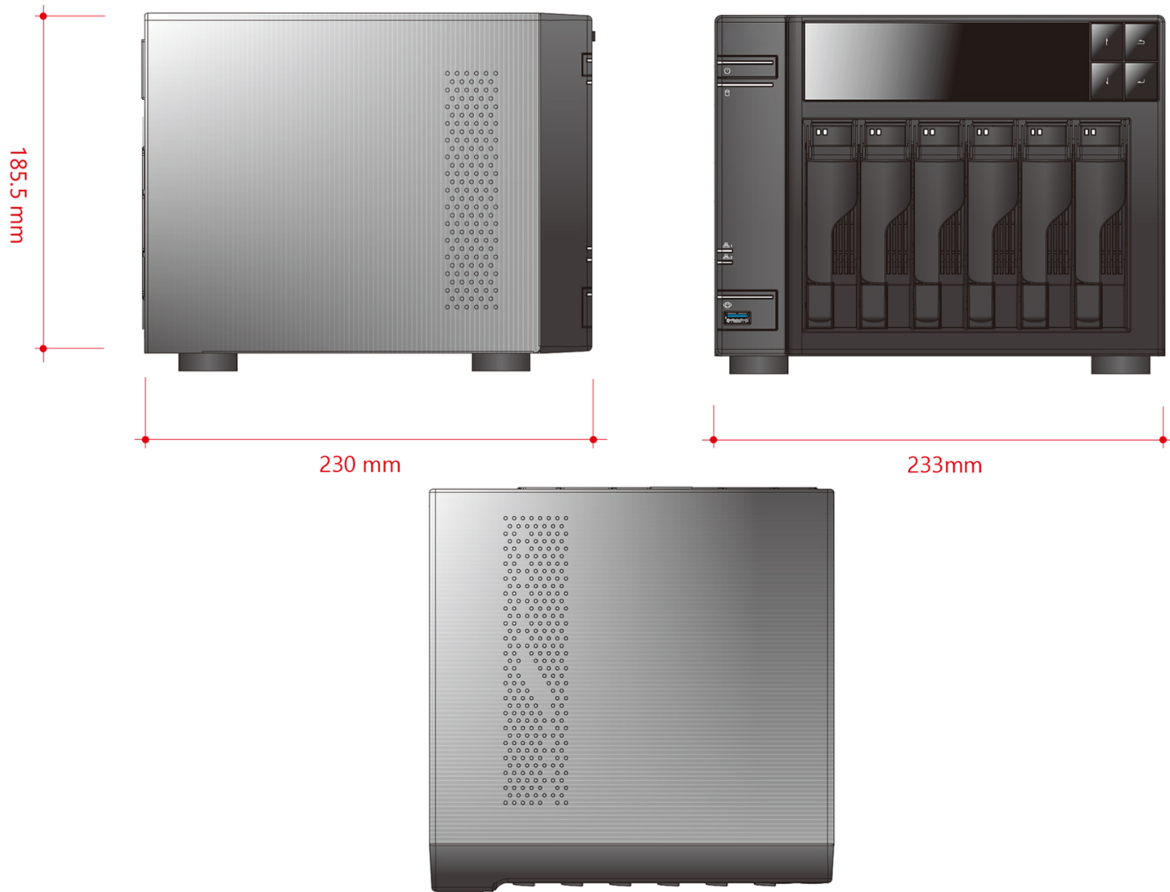
NVR-Pro-T64-A6 製品寸法図
